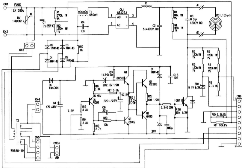
格兰仕 IMP1, HYP1 系列电磁炉功率输出板电路图
