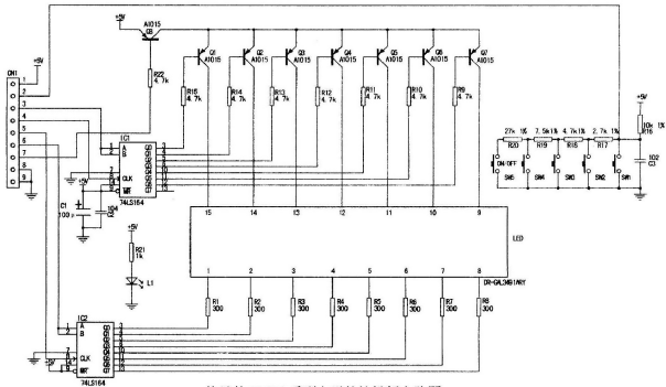
格蘭仕 HYP1 系列电磁炉按键板电路图
