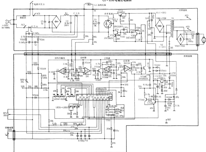
CY-1330 电磁灶电路图
