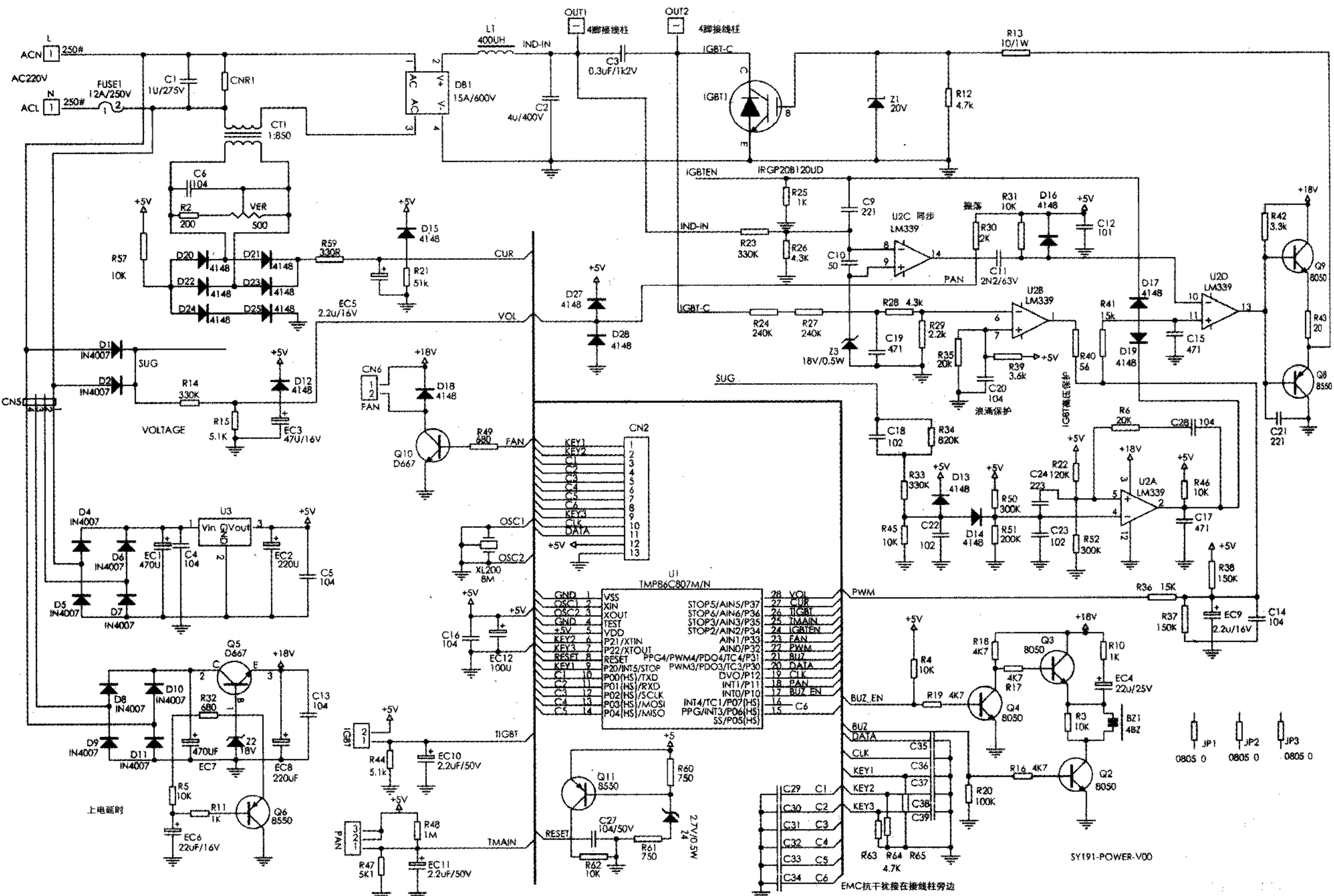
美的 SY191 型电磁炉主板电路原理图
